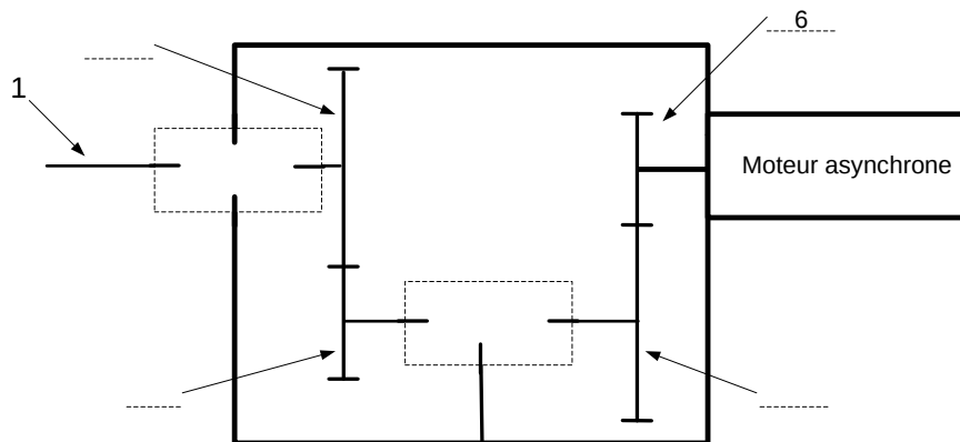
Schéma cinématique à compléter
